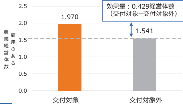
図2 分析例：平均的な介入効果
